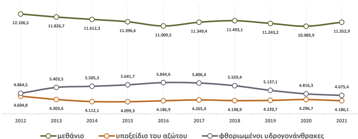
Γράφημα 6. Εκπομπές του μεθανίου ( CH_4 ), του υποξειδίου του αζώτου ( N_2O ) και των φθοριωμένων υδρογονανθράκων (HFCs) σε 1.000 τόνους ισοδύναμου CO_2 , 2012 – 2021*
