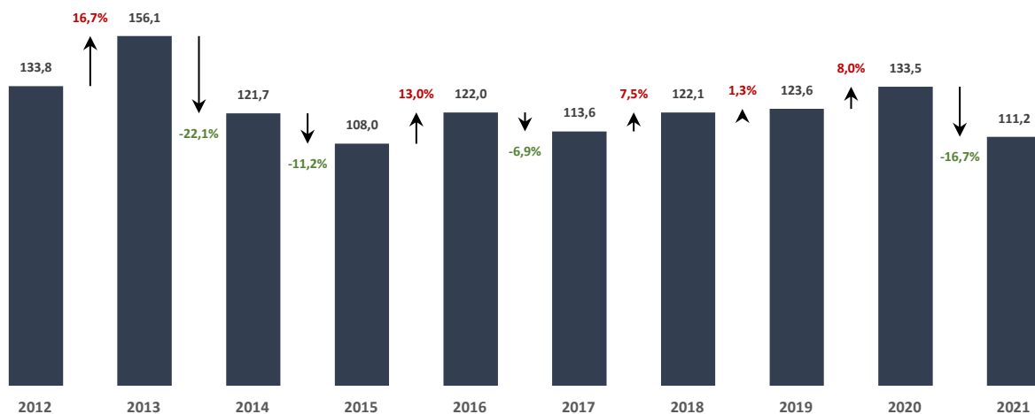
Γράφημα 7: Εκπομπές των υπερφθορανθράκων (PFCs) σε 1.000 τόνους ισοδύναμου CO 2 και ετήσια ποσοστιαία μεταβολή (%), 2012 – 2021*
