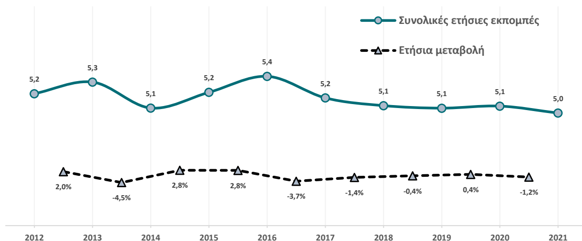
Γράφημα 8: Εκπομπές του εξαθφοριούχου θείου (SF 6 ) σε 1.000 τόνους ισοδύναμου CO 2 και ετήσια ποσοστιαία μεταβολή (%), 2012 – 2021*
