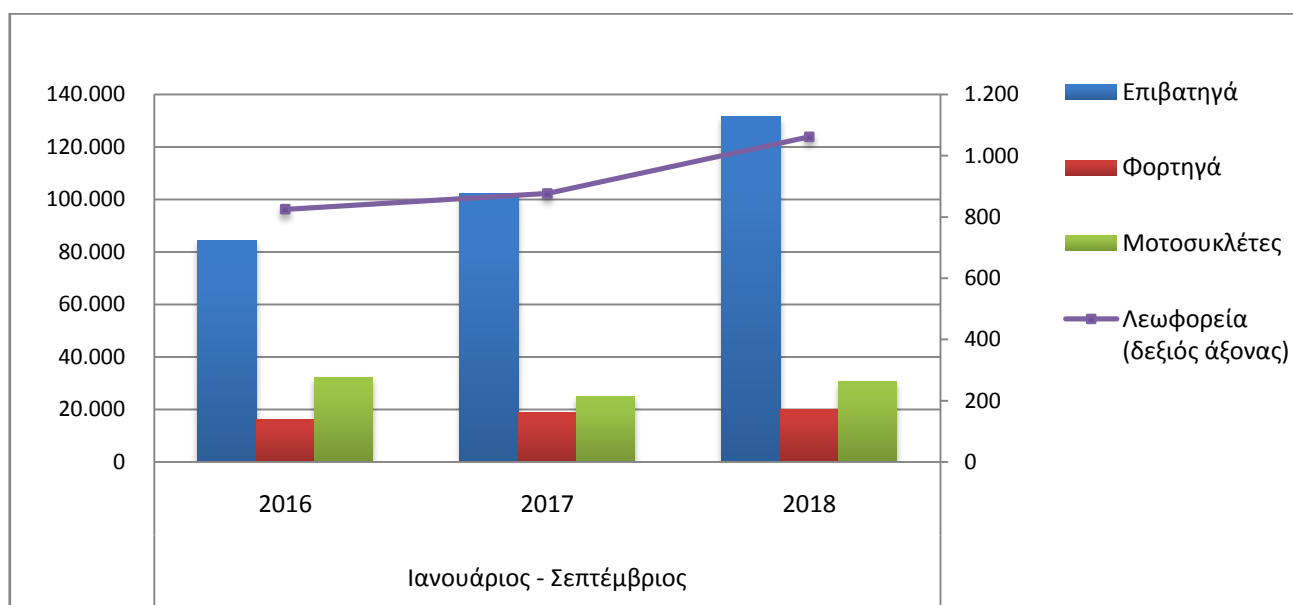
Γράφημα 7. Νέες Εγγραφές Οχημάτων : Ιανουάριος - Σεπτέμβριος 2018
